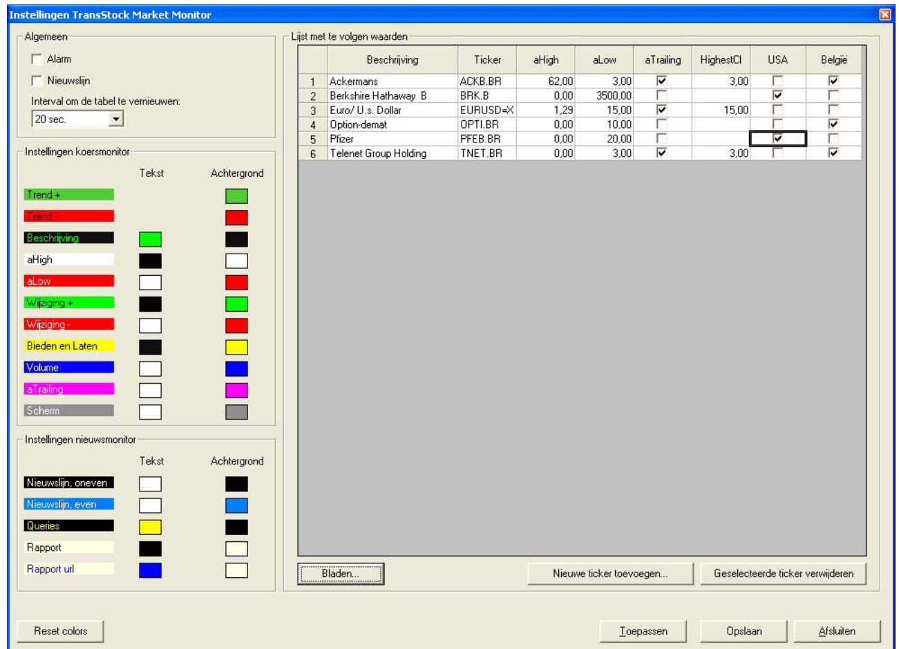
Figuur 8: Het venster waarmee de instellingen van de MM geregeld worden.
